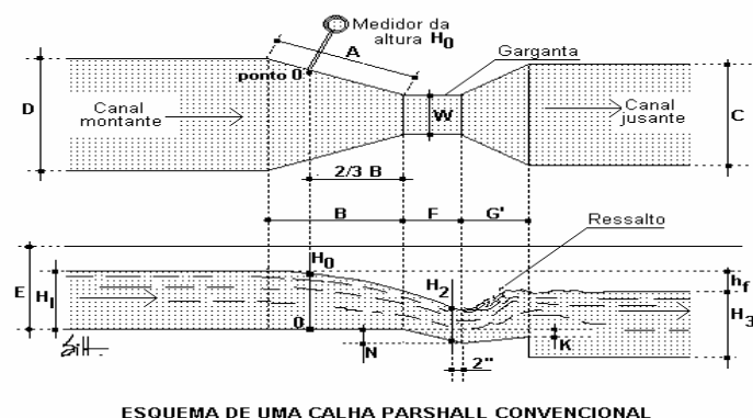
Figura 1. Detalhes do medidor de regime crítico denominado calha Parshall
